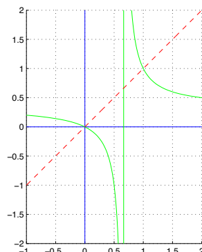
Figura 17: Esercizio 19 g(x)
