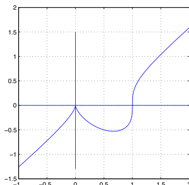
Figura 16: Esercizio 19 f(x)
