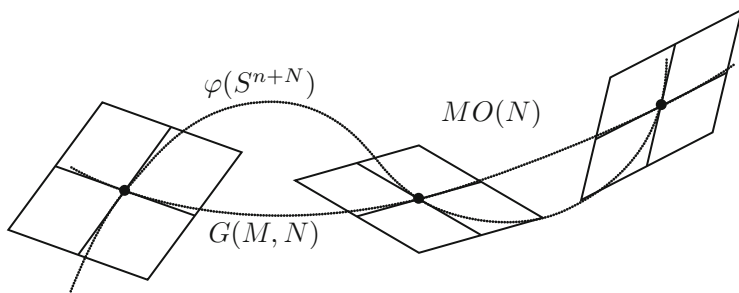
Fig. 139 t -regular map
