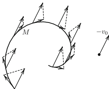
Fig. 137 Computing \text{deg}(S^n \rightarrow S^n)
