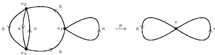
Figura 12.3. Un rivestimento dell'otto.
