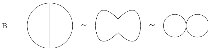
Figura 10.1. Sottoinsiemi del piano con forme equivalenti.
