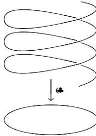
Figura 12.1. Identificando \mathbb{R} con l'elica regolare E = \{(z, t) \in \mathbb{C} \times \mathbb{R} \mid z = e(t)\} tramite l'omeomorfismo t \mapsto (e(t), t) , il rivestimento e: \mathbb{R} \rightarrow S^1 coincide con la restrizione all'elica della proiezione p: \mathbb{C} \times \mathbb{R} \rightarrow \mathbb{C} .
